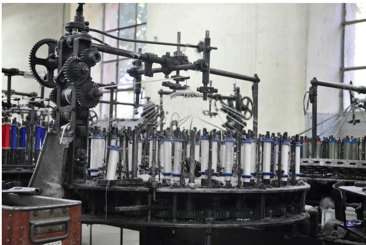
Métier à tresser métallique
