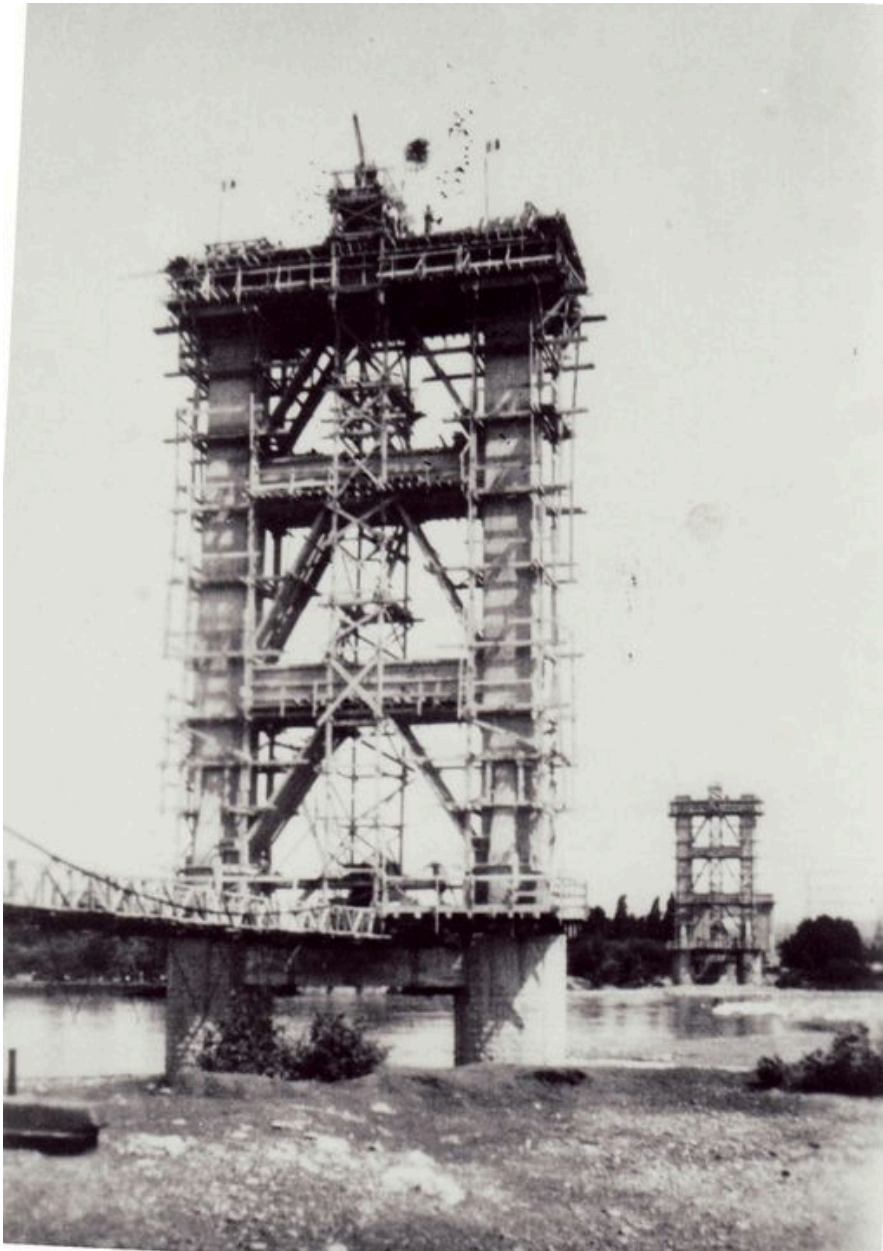
[Reconstruction du pont - les pylônes] / Cheynet phot. Le Teil : Cheynet, [ca 1948]. 1 photogr. pos. : n. et b. (Lyon, Inventaire général)
