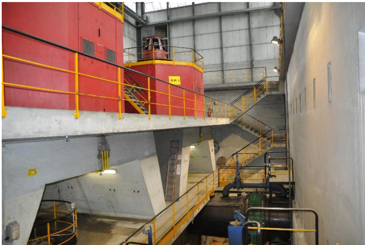
Vue de deux groupes verticaux dans la salle des machines
