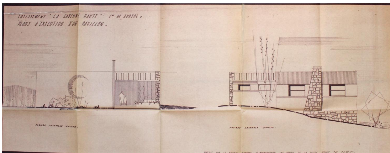
Durtol, la maison B., façades latérales, Roger Bourgougnon maître d'œuvre, 1964 (archives municipales de Durtol).
