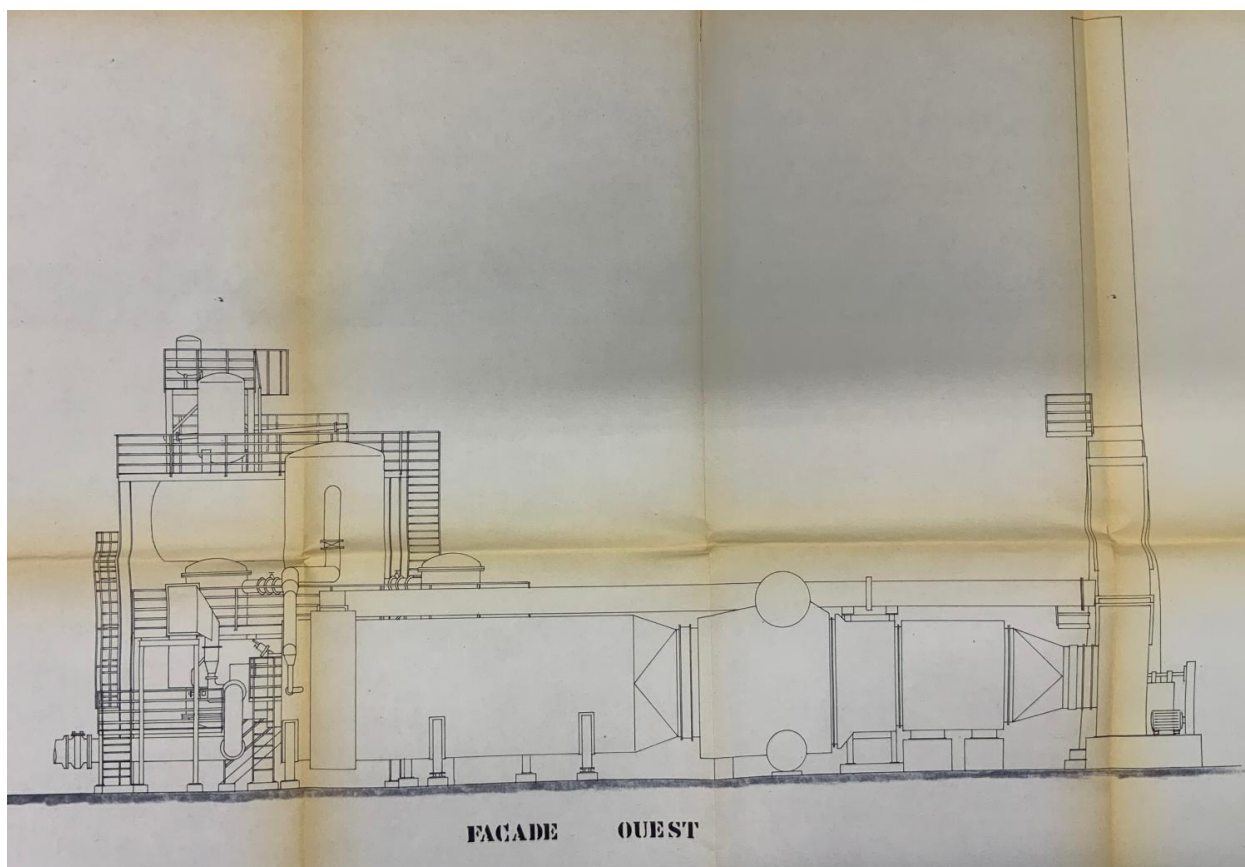
Plan incinérateur de sous-produits, architecte Gérard Senglet, 1981 (AC Pierre-Bénite : 203 – 81)
