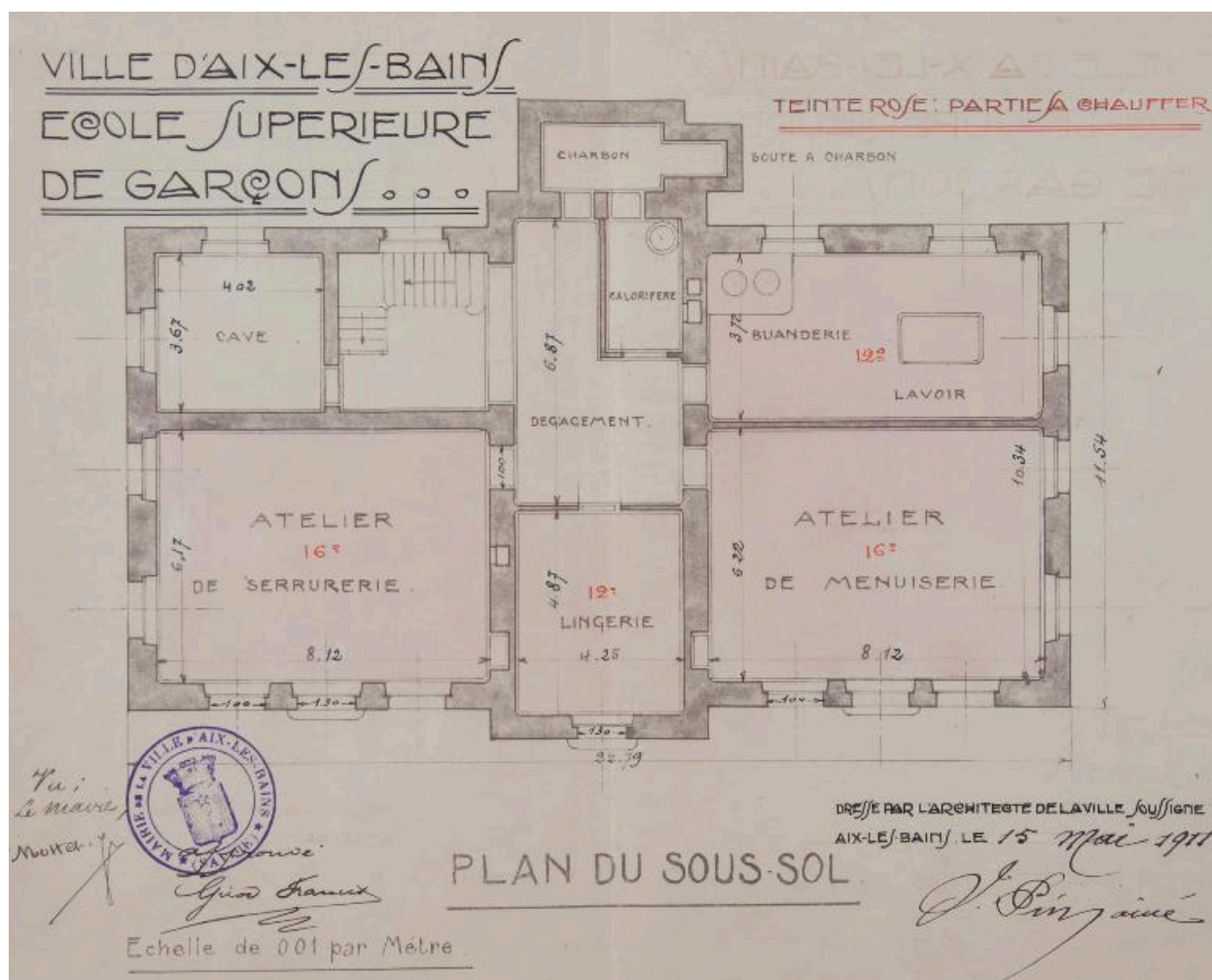
Plan du sous-sol, 1911
