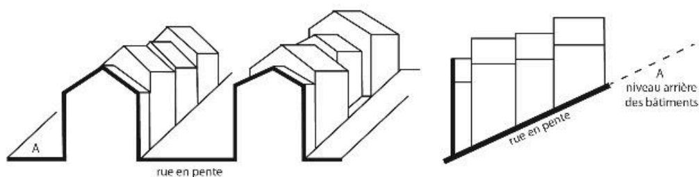
Coupes sur rue parallèle à la pente
