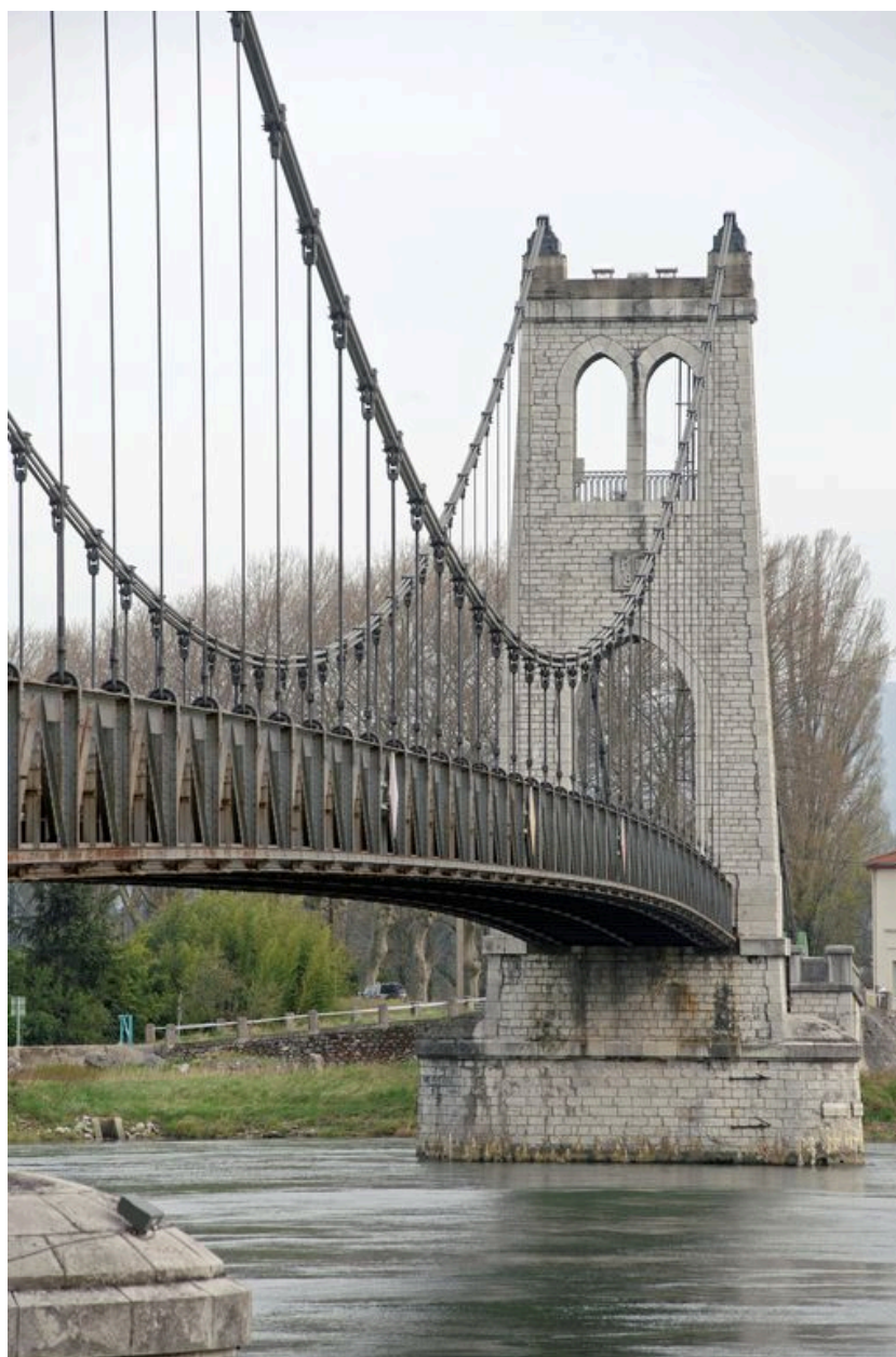
Vue côté aval (depuis la rive droite)
