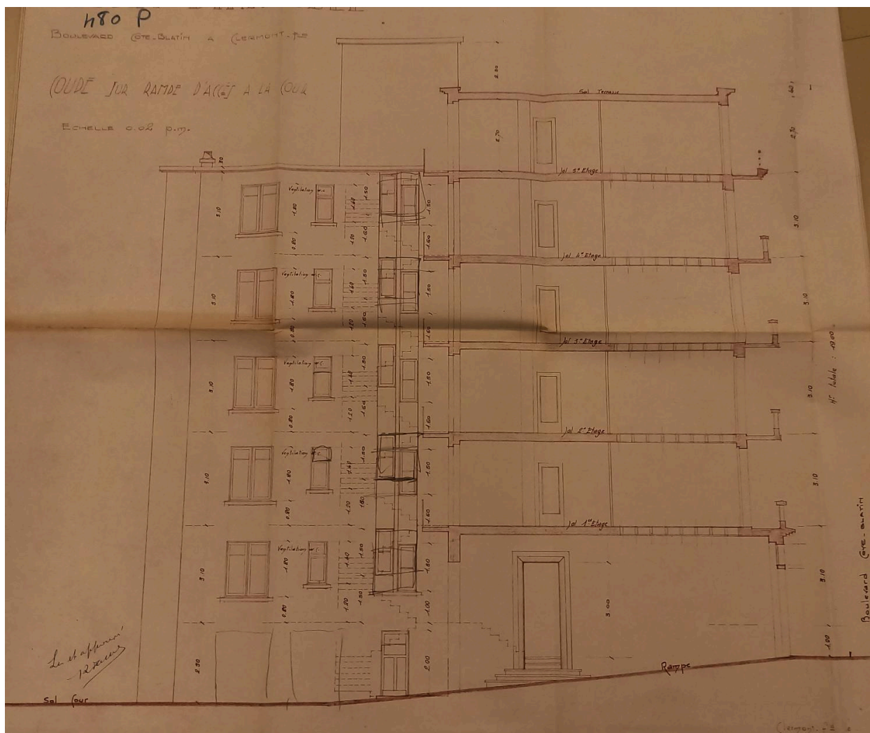
Coupe longitudinale
