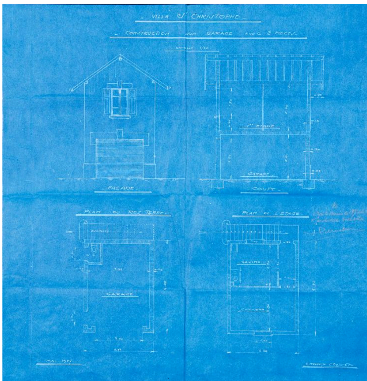
Garage et logement, plans, 1927
