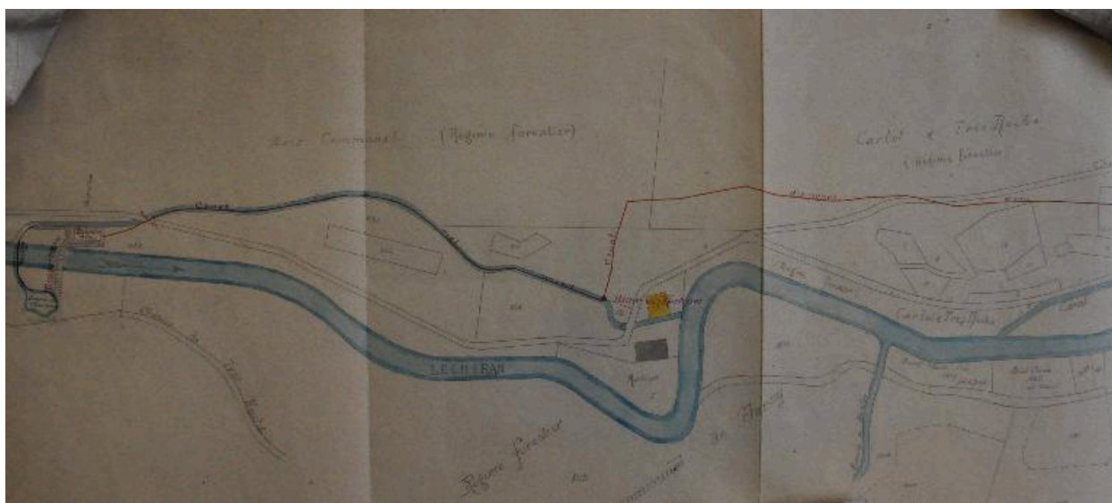
Plan concernant le projet de transformation du moulin en centrale hydroélectrique, vue 1, 1919 (FR.AD073, 81S42).
