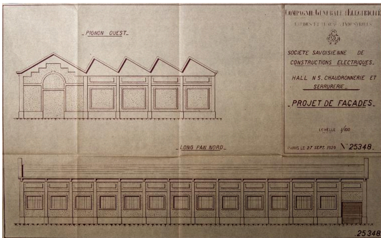
Projet de façade pour la halle de chaudronnerie, 1929
