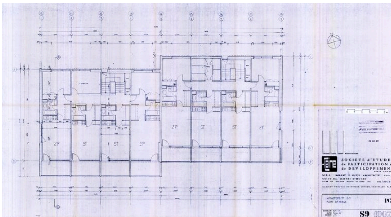
Plan 3e étage. M.B.A. Robert K Gatje architecte, CO.TE.BA. maître d'oeuvre, 5 avril 1977 (AC Arâches-la-Frasse)
