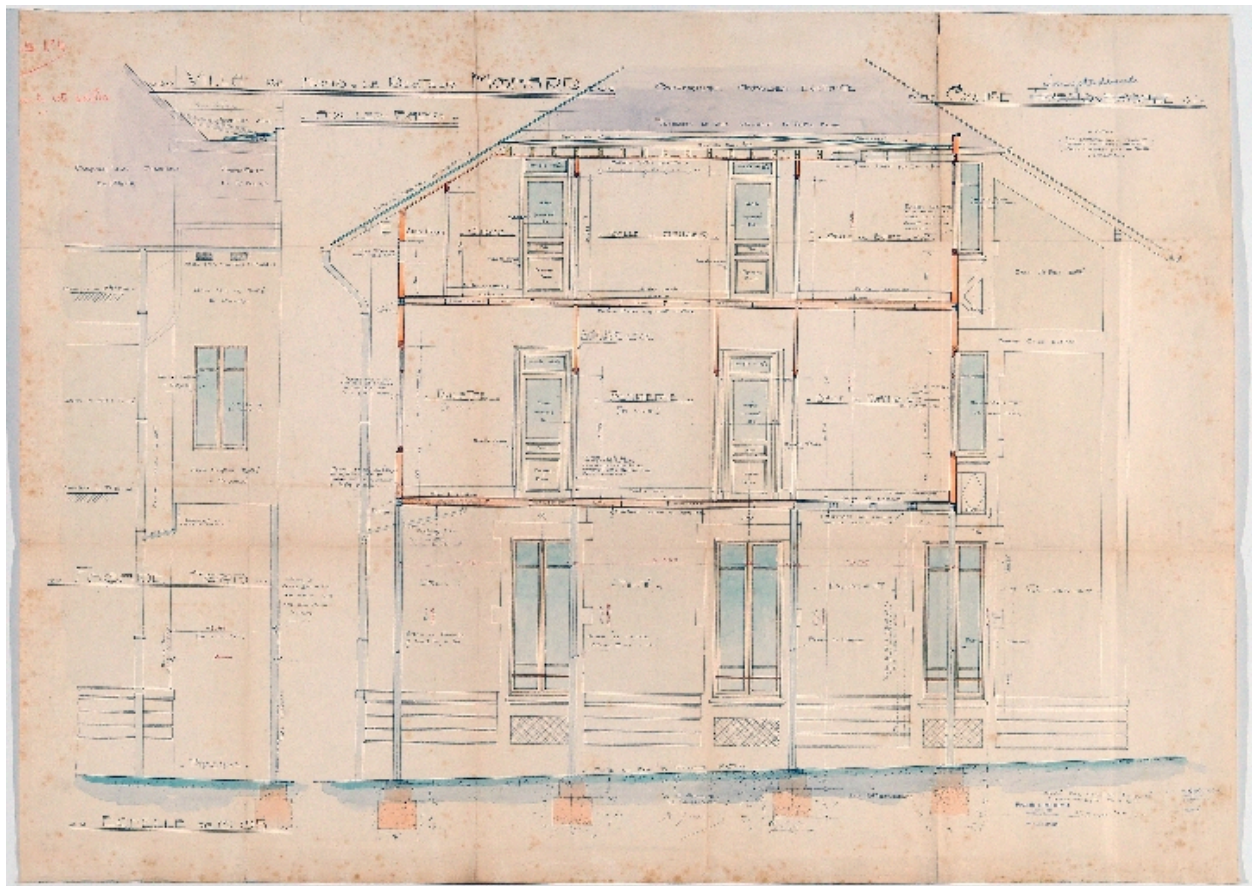
Coupe et élévation du corps de porche droit
