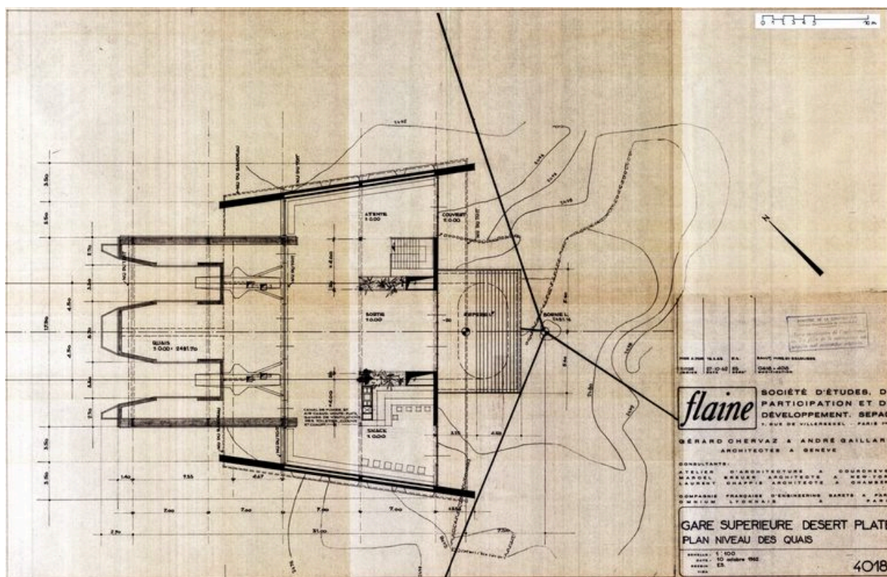
Plan au niveau des quais. Gérard Chervaz et André Gaillard architectes, 10 octobre 1962. Modifié les 27 octobre 1962 et 18 février 1963 (AC Magland)
