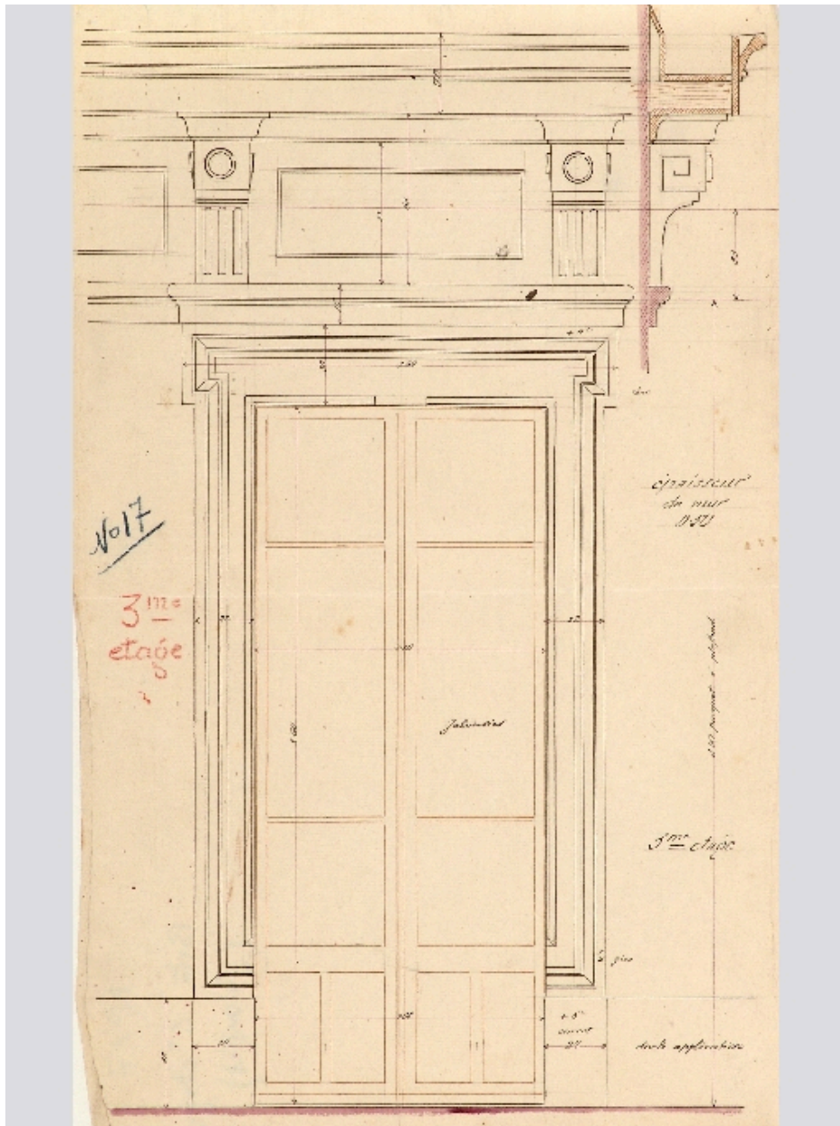
Détail de l'élévation du 3e étage
