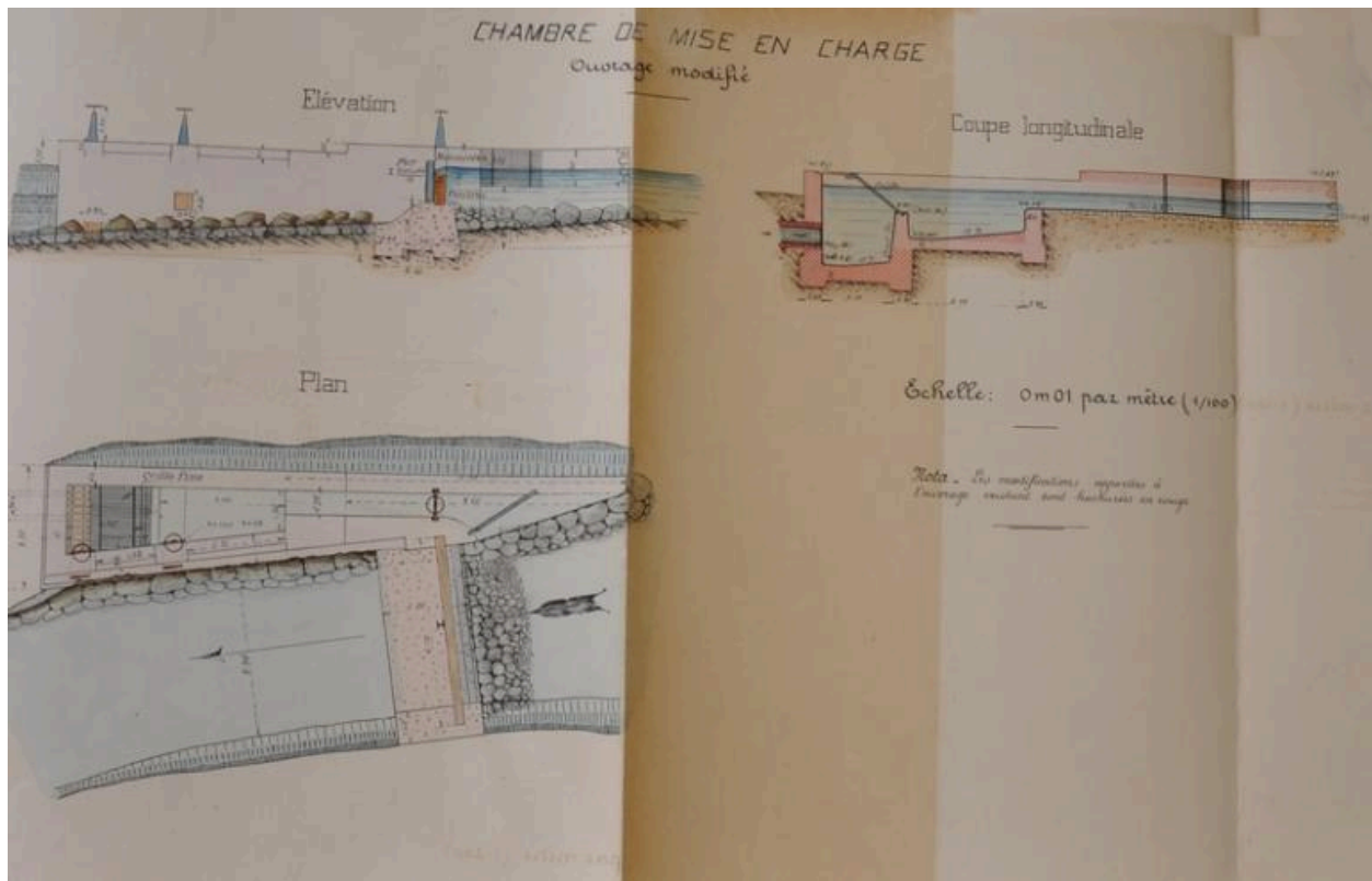
Plan accompagnant la demande de construction de la centrale, 1921 (FR.AD073, 83S28).
