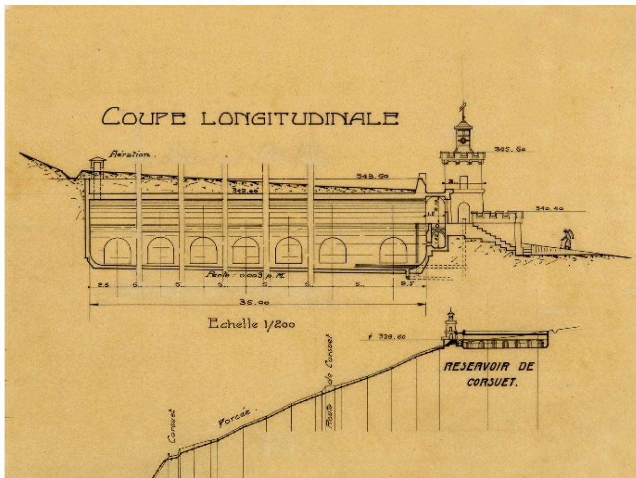
Coupe longitudinale
