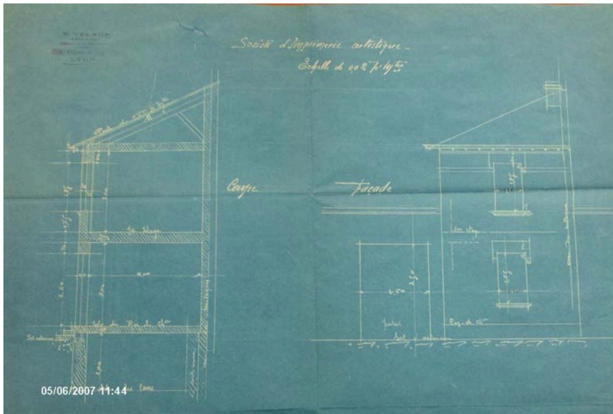
Façade et coupe 1907 : Sté IAC ; construction d'un loge de gardien
