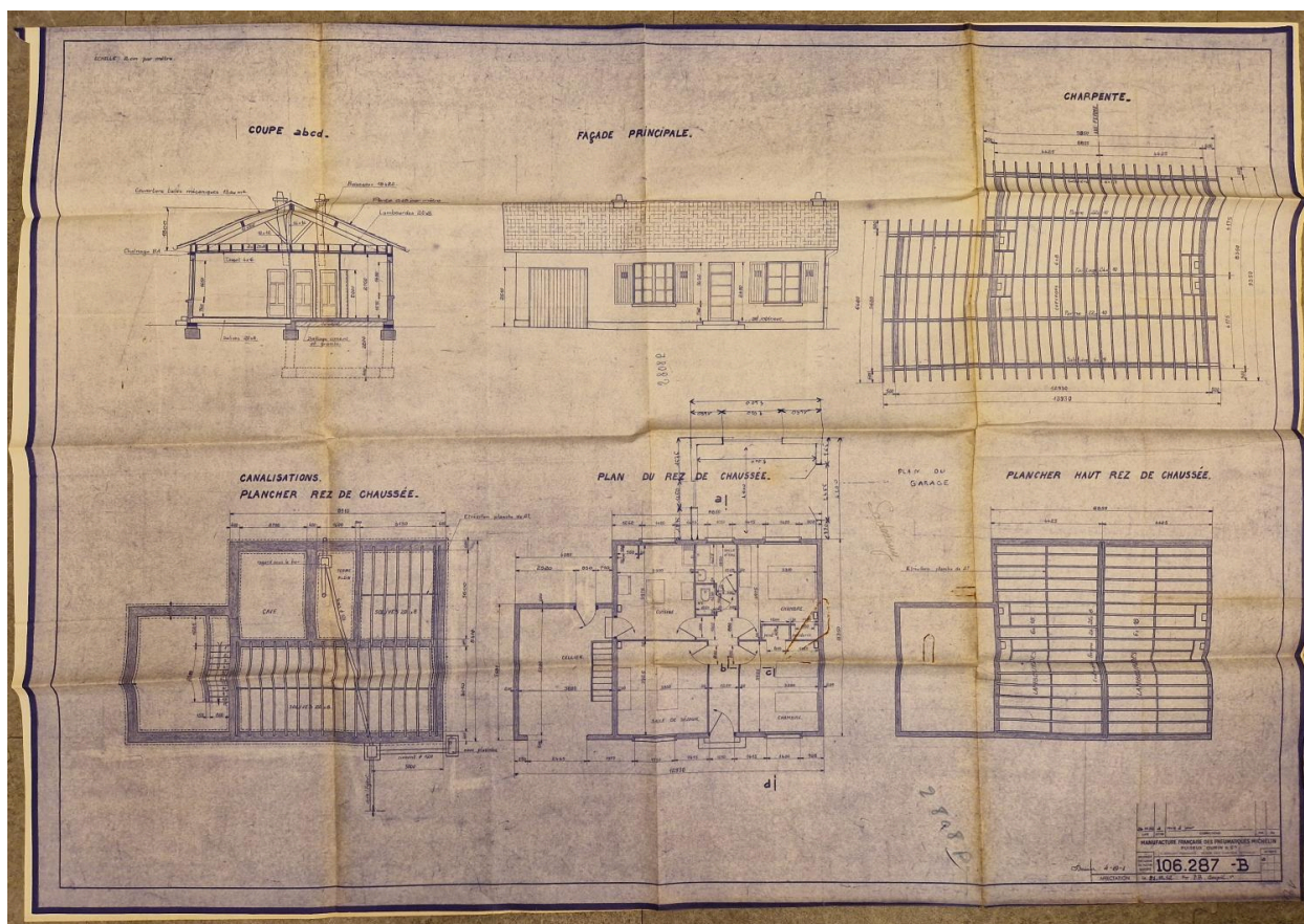
Plans, coupe et élévations d'une habitation "Castor" en rez-de-chaussée (2e modèle), allée des Castors, 1952.
