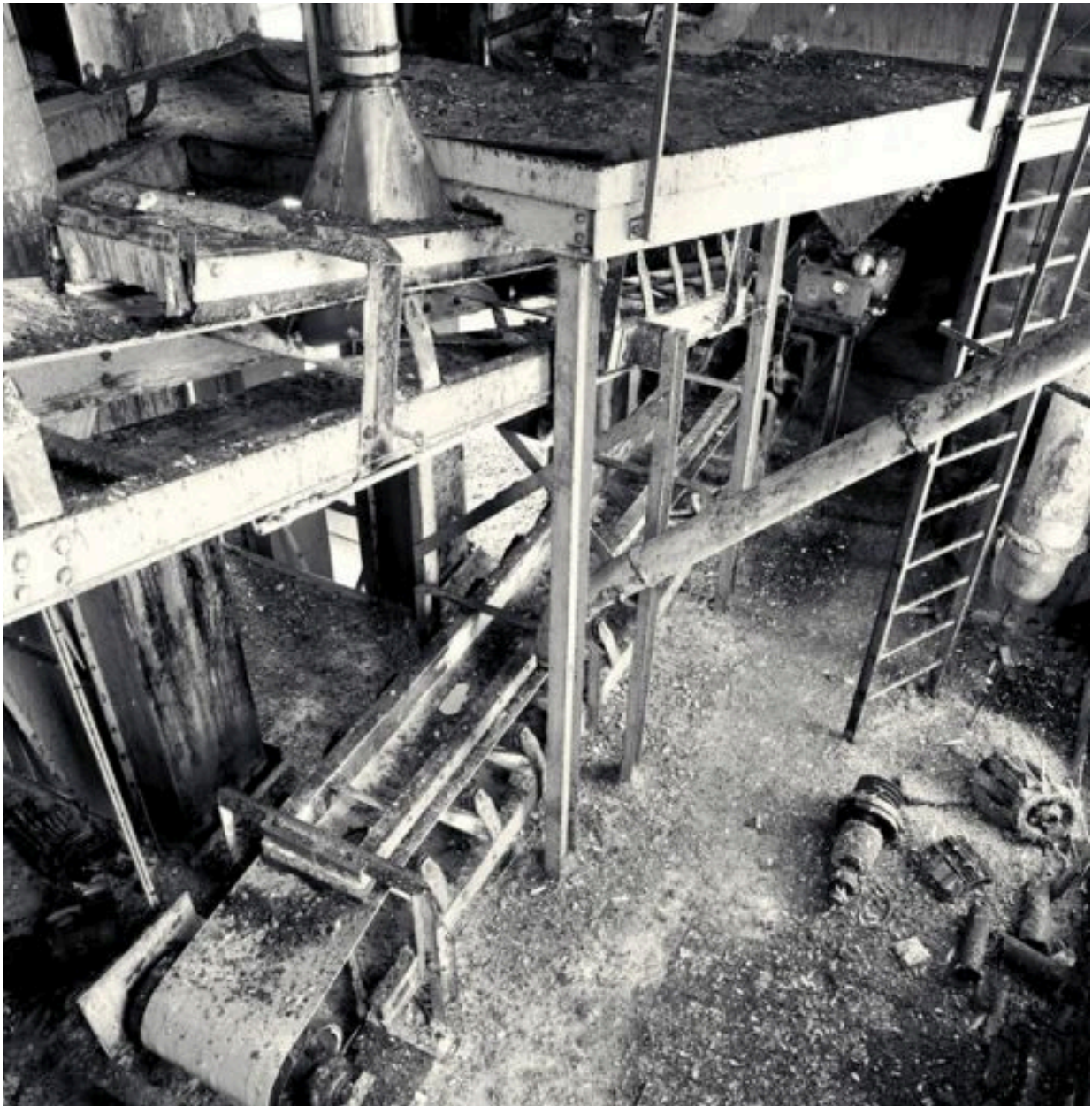
La cage des élévateurs : jonction des transporteurs à bandes
