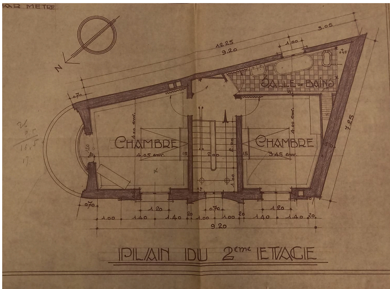
Plan du deuxième étage
