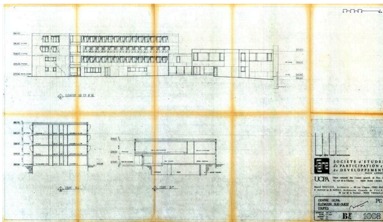
Elévation sud-ouest et coupes. Marcel Breuer architecte, R. Jahan et R. Sadoli architectes conseils de l'UCPA, 9 juillet 1975 (AC Magland)
