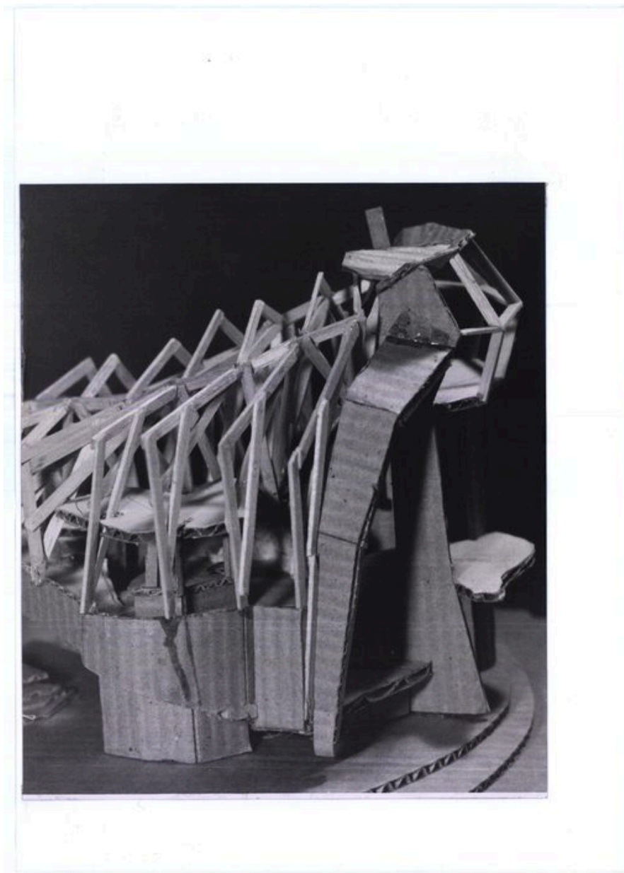
Maquette d'étude en carton. Détail de charpente / J. Labro (A. privées J. Labro)
