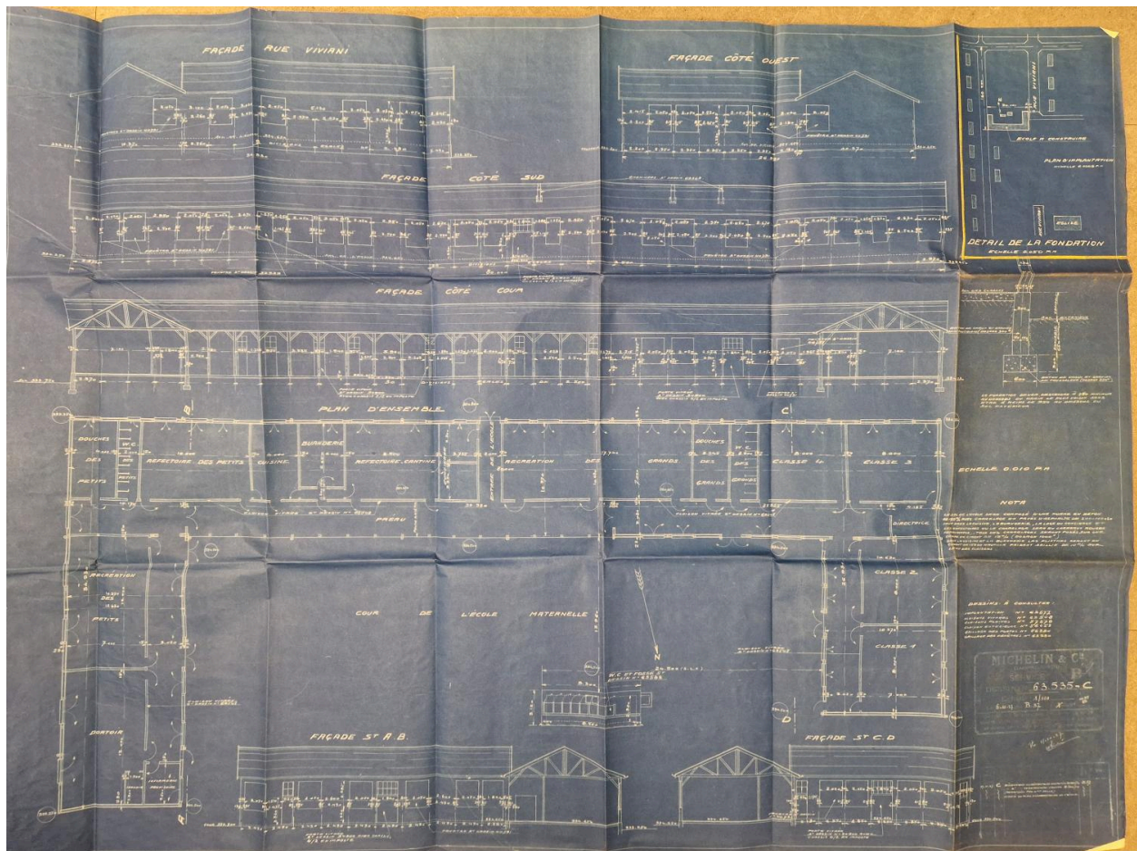
Projet de groupe scolaire à la Plaine, rue Viviani (école Mercœur) : plan, coupes, élévations, 1927.
