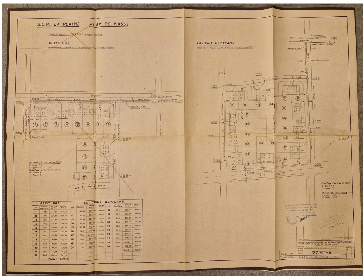
Projet de lotissement rue Rouvier (quartier de la Croix-Bertrand) : plan masse, 1961.
