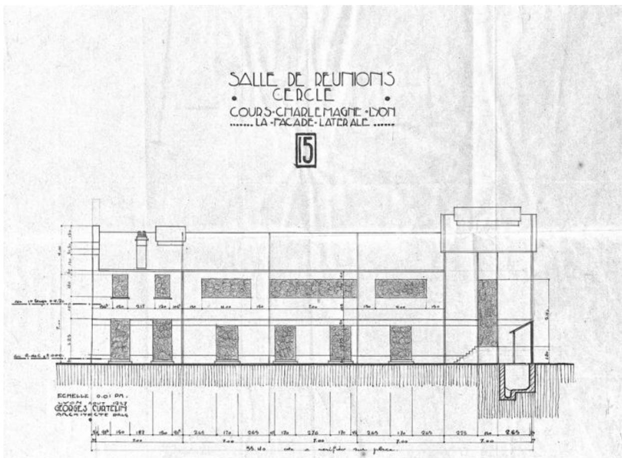
Elévation latérale
