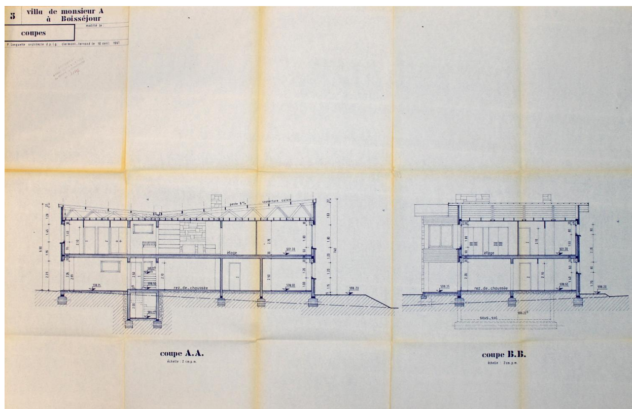
Ceyrat, la maison A., coupes, Paul Lanquette architecte, avril 1967 (archives départementales du Puy-de-Dôme).
