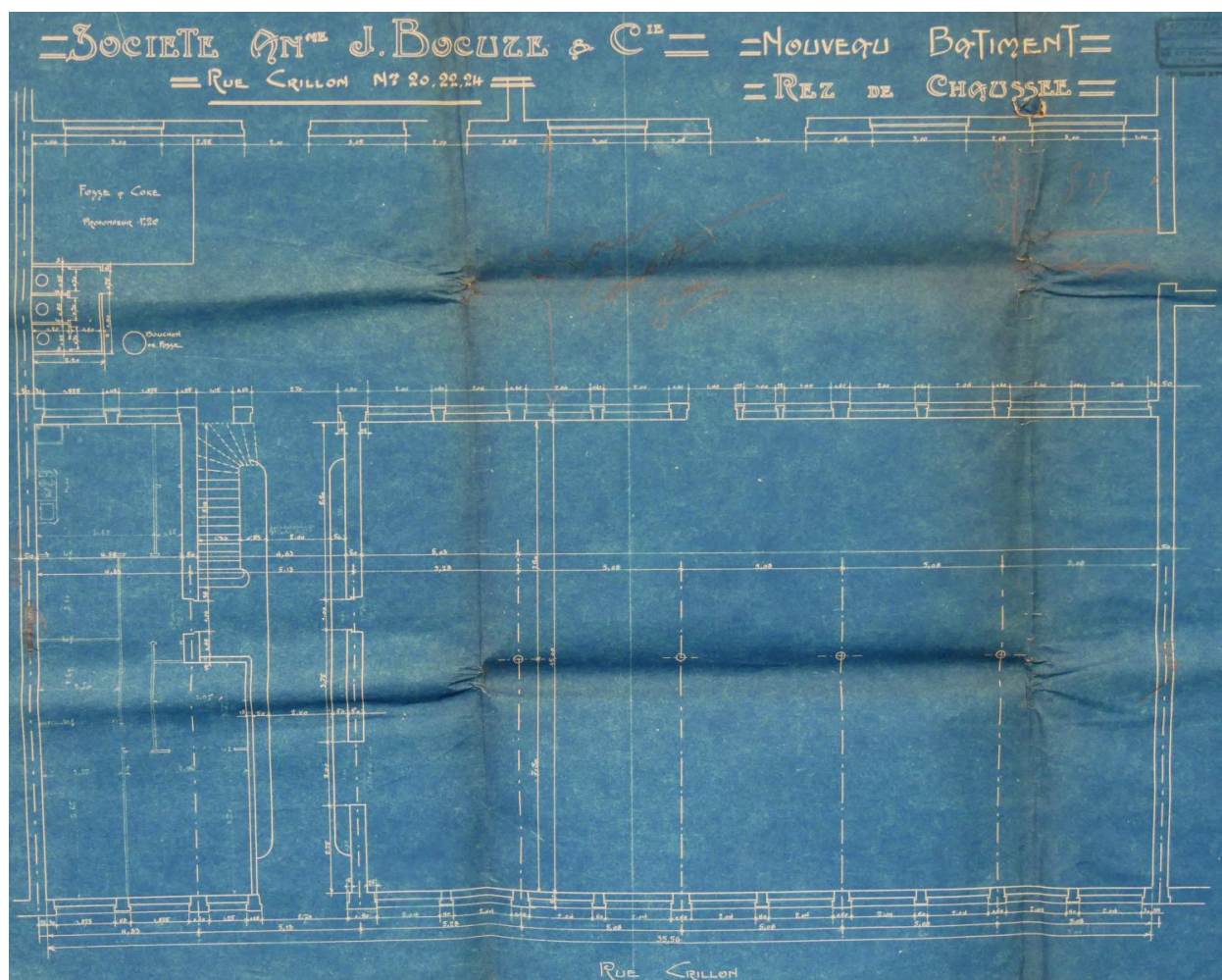
Rez-de-chaussée usine Bocuze (AC Lyon 314W/480)
