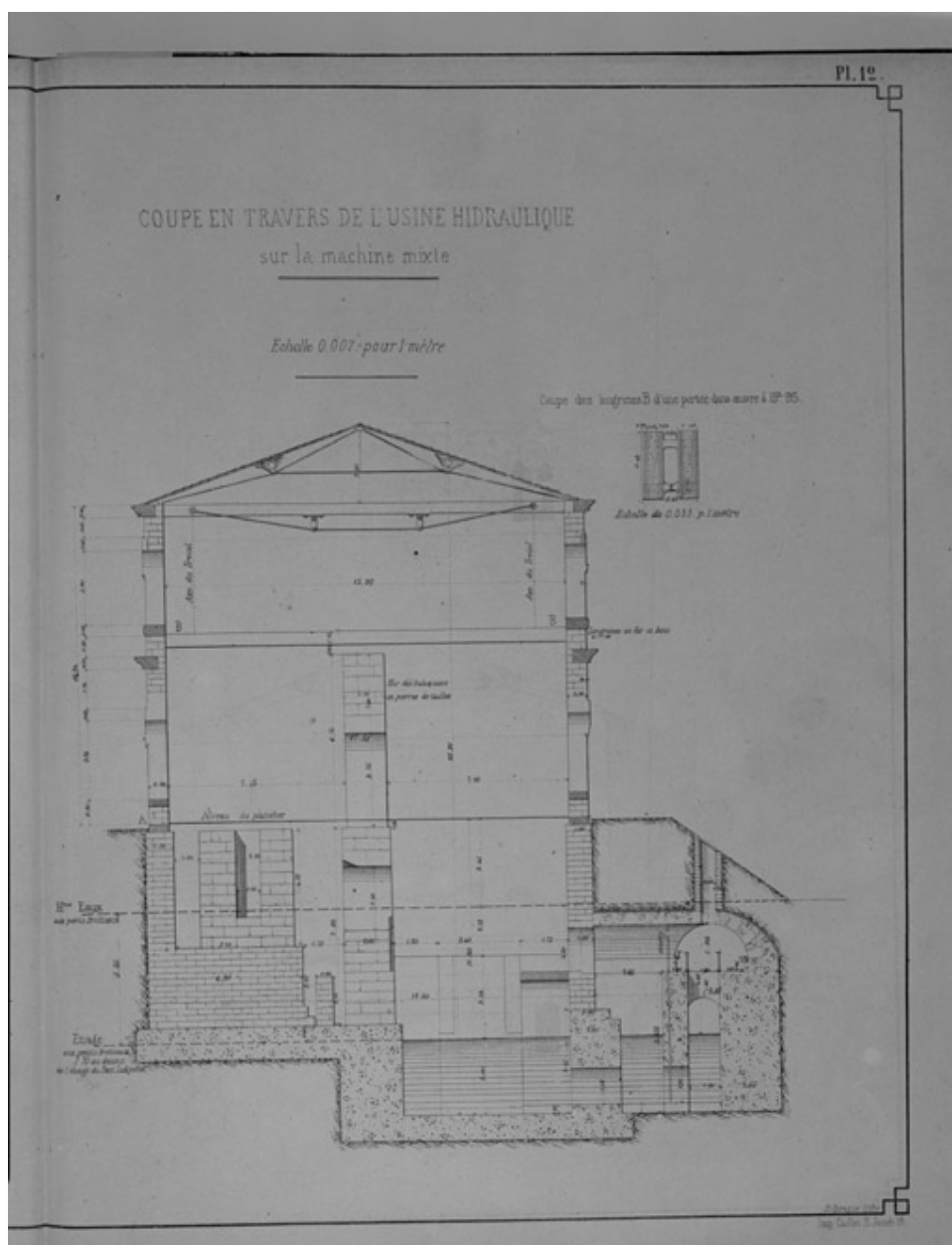
Coupe en travers de l'usine hydraulique
