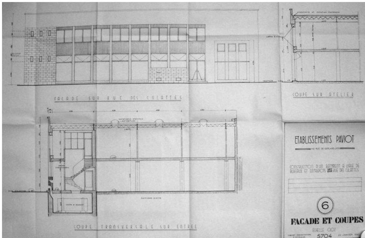
Façade sur rue Marcel Mérieux et coupes, 255 rue des Culattes, 20 janvier 1961 par Pierre Renaud architecte, échelle 1/50. (Arch. mun. Lyon)
