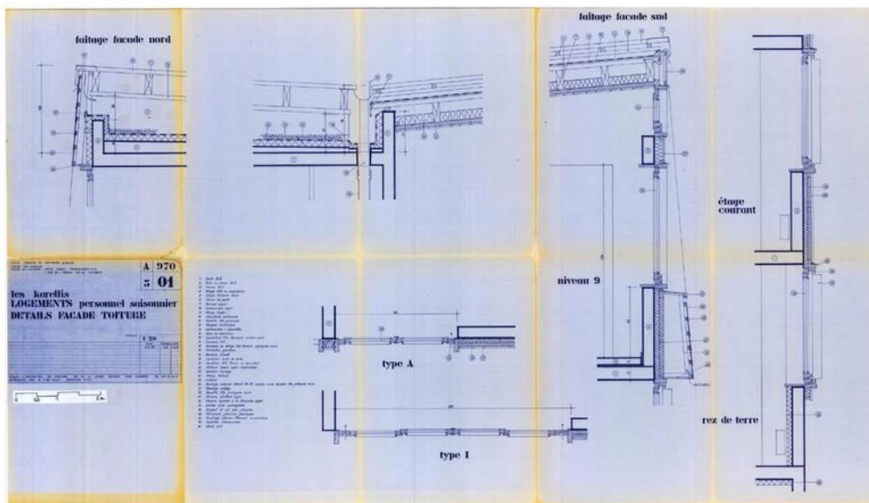
Logements personnel saisonnier. Détails de façade et de toiture / Atelier d'architecture en Montagne, 9 mars 1978. Modifications 22 juin 1979 (AC Montricher-Albanne)
