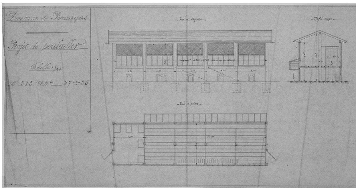
Domaine de Beaurevers. Projet de poulailler. 27 mars 1925.
