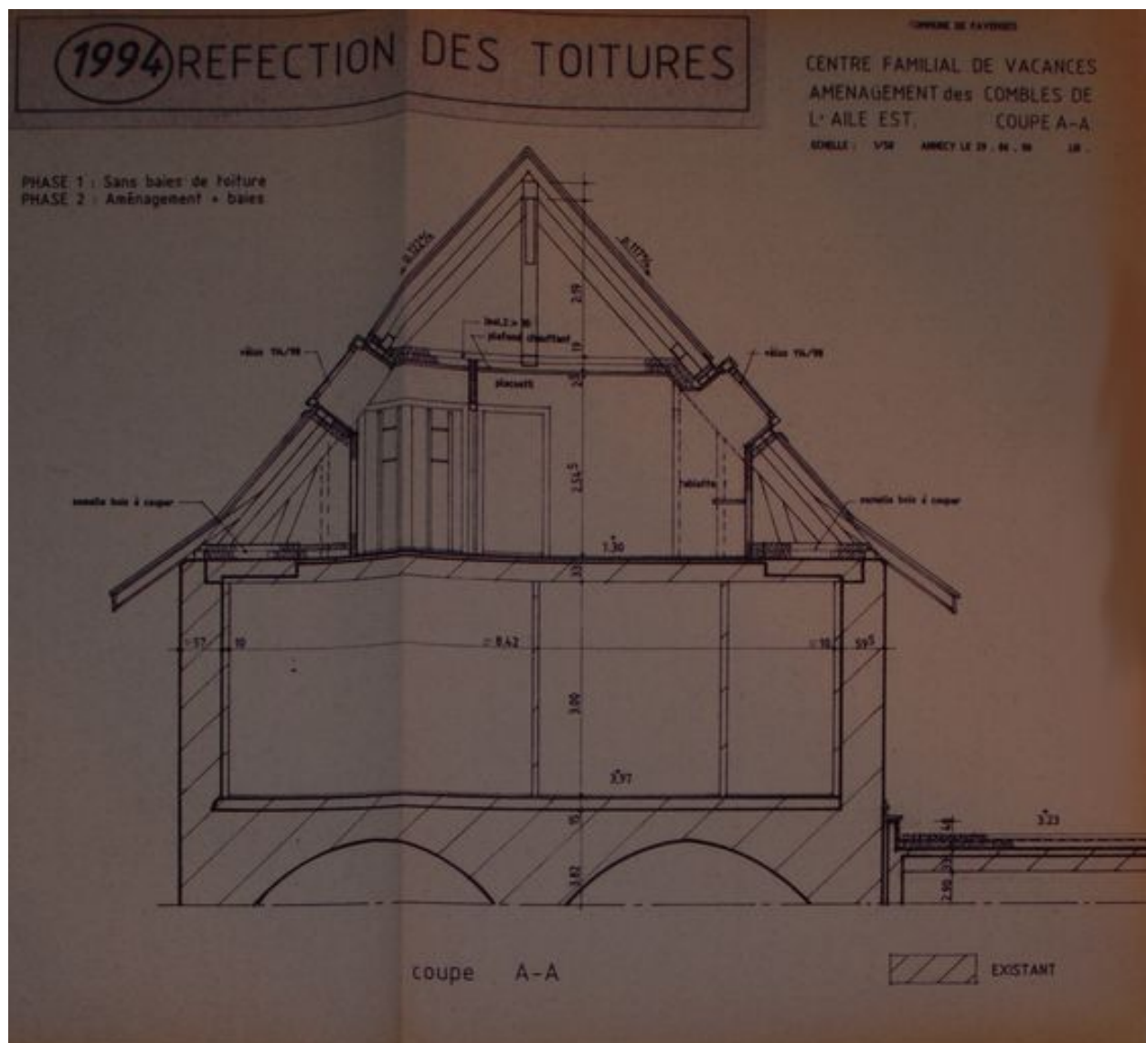
Aile est, coupe A-A des combles, 29 juin 1994. Plan. Archives municipales de Faverges © Archives municipales de Faverges. 5 Fi 34/10
