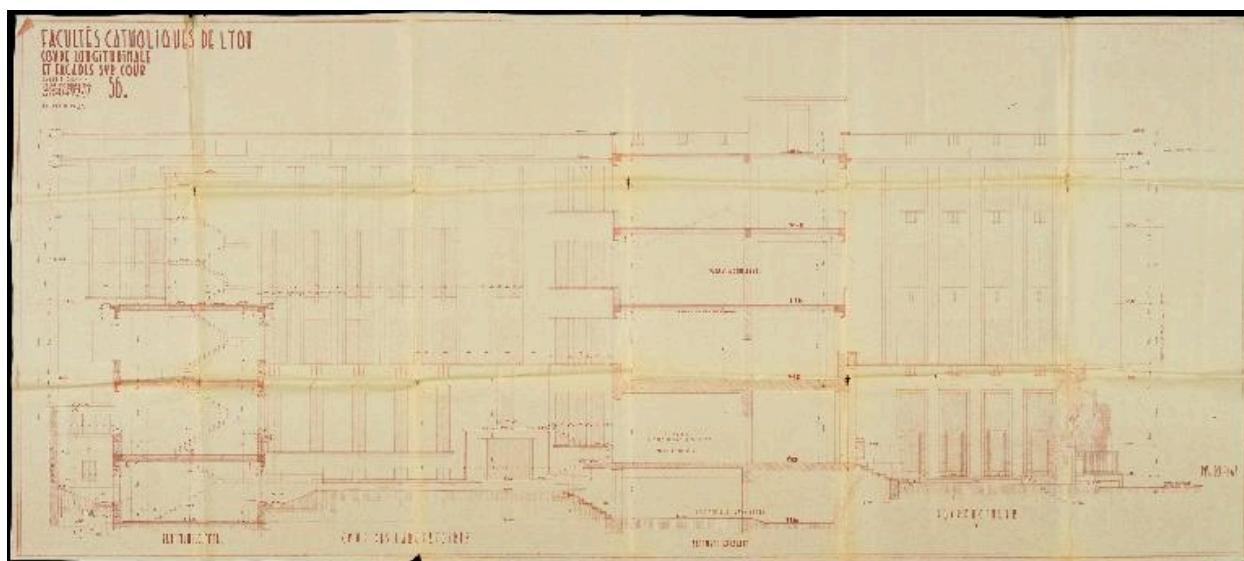
plan façade sur cour et coupe longitudinale par G. Curtelin, 1938
