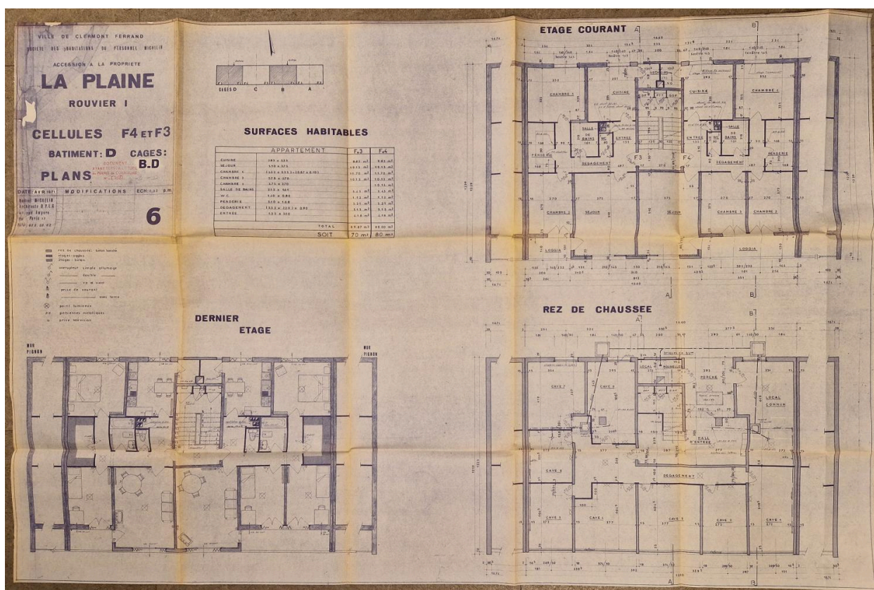
Projet d'immeubles collectifs, rue Rouvier : plans du rez-de-chaussée, des étages courants et du dernier étage du bâtiment D (cages B et D), 1971.
