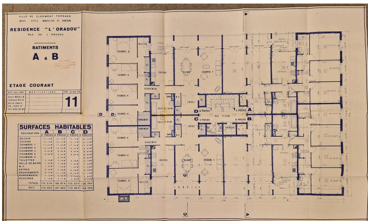
Projet de résidence "l'Oradou" : plan de l'étage courant des bâtiments A et B, 1971.
