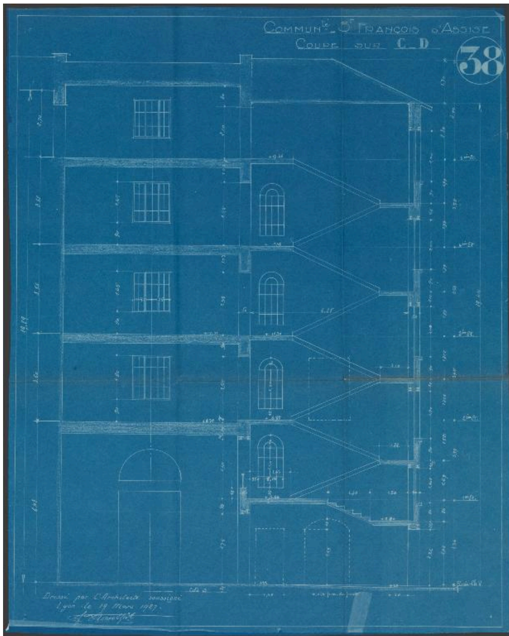
Communauté Saint-François d'Assise : coupe sur CD / François Roux-Spitz architecte. 1927 (AC Lyon 344 W 732)
