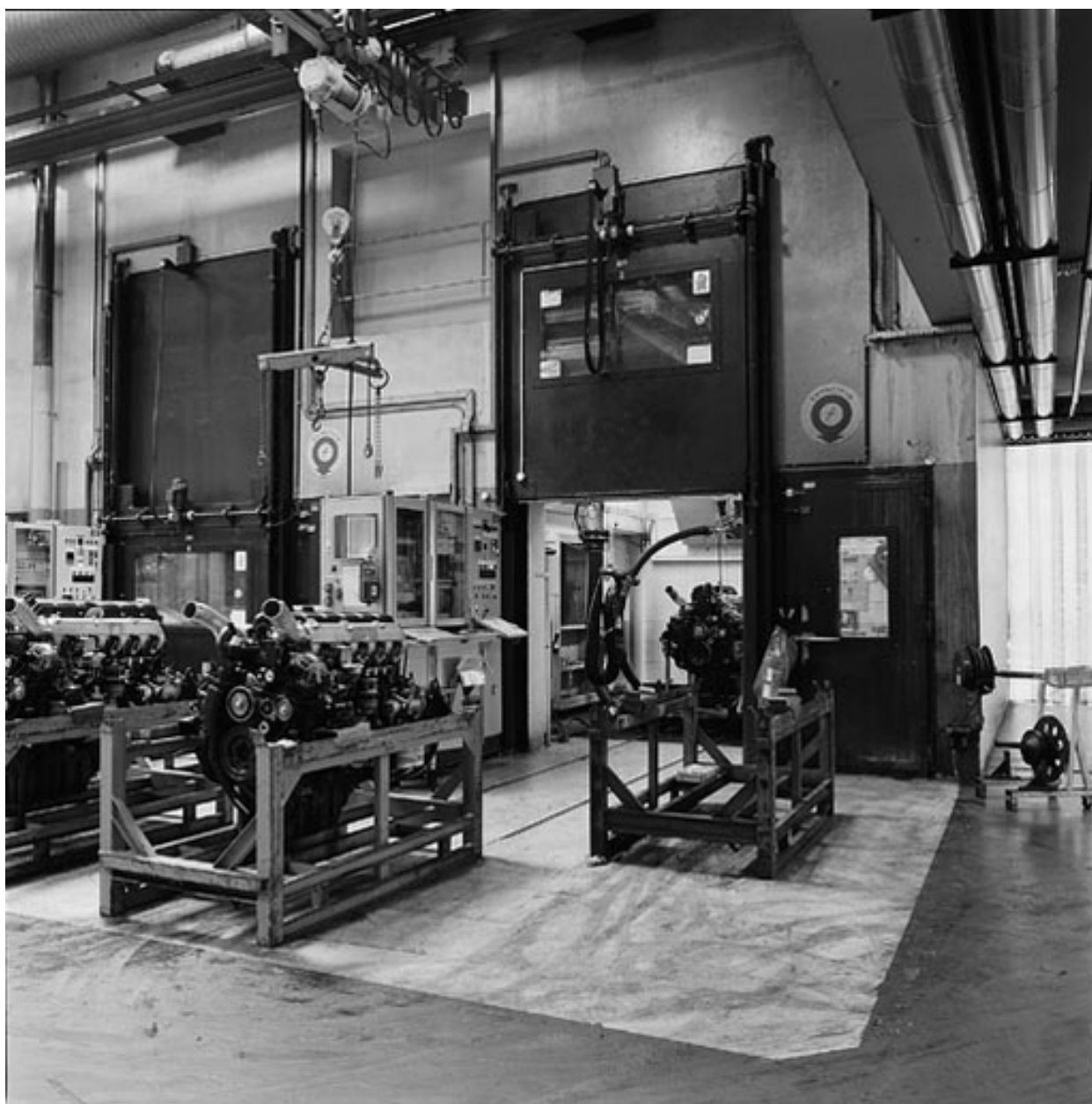
Usine moteur : cellule essai moteur.
