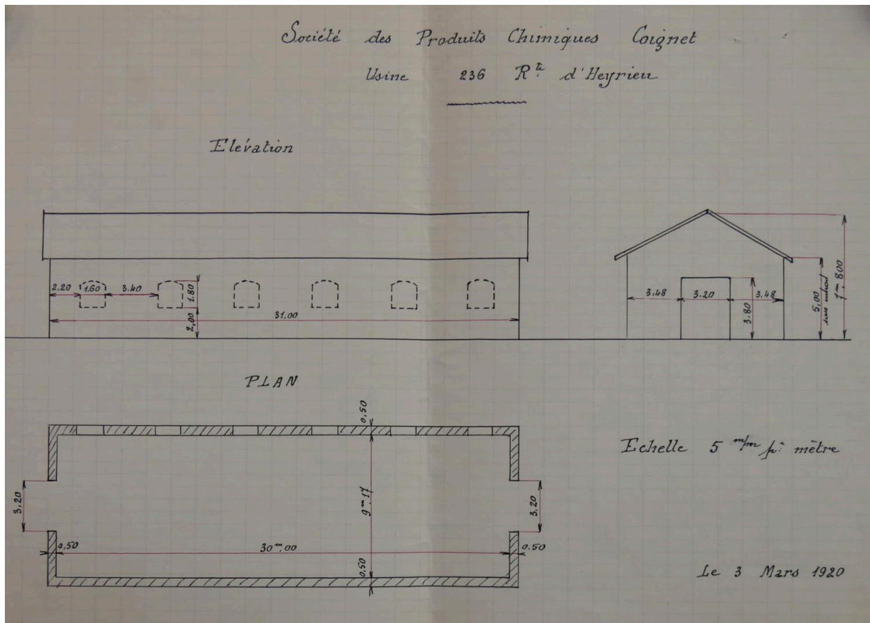
Bâtiment des chlorures élévation, usine chimique Coignet 1920 (ACL 314W 357)
