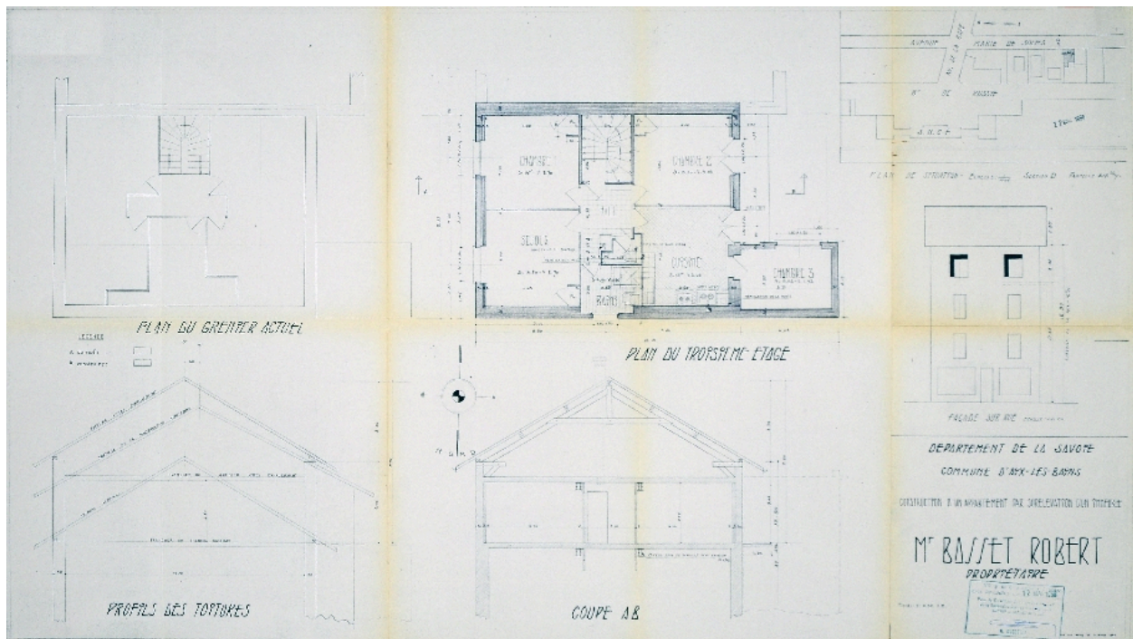
Plans, élévation et coupes
