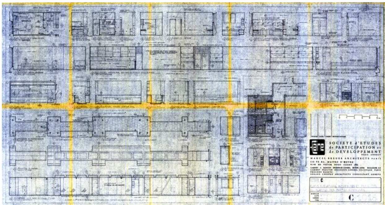
Hôtel C. Plan, élévations intérieures et projection du plafond des parties communes. Marcel Breuer architecte, 30 octobre 1967 (AC Arâches-la-Frasse)
