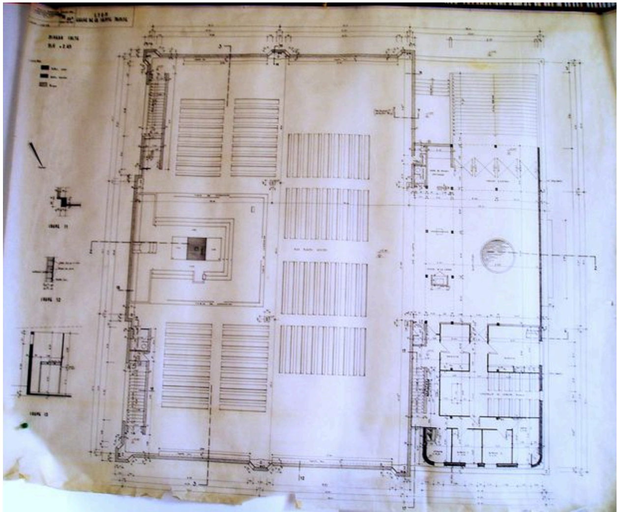
Plan du niveau du culte, par P. Genton, février 1961 (AP Société académique d'architecture de Lyon)
