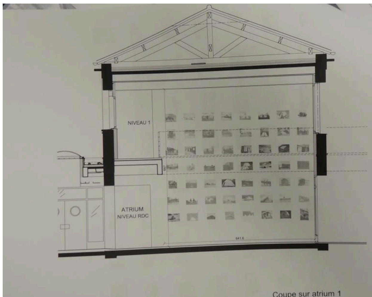
Coupe sur atrium 1.
