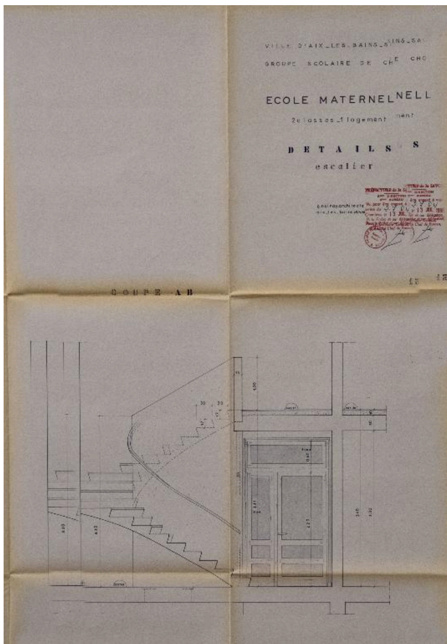
Détail de l'escalier, coupe, 1966
