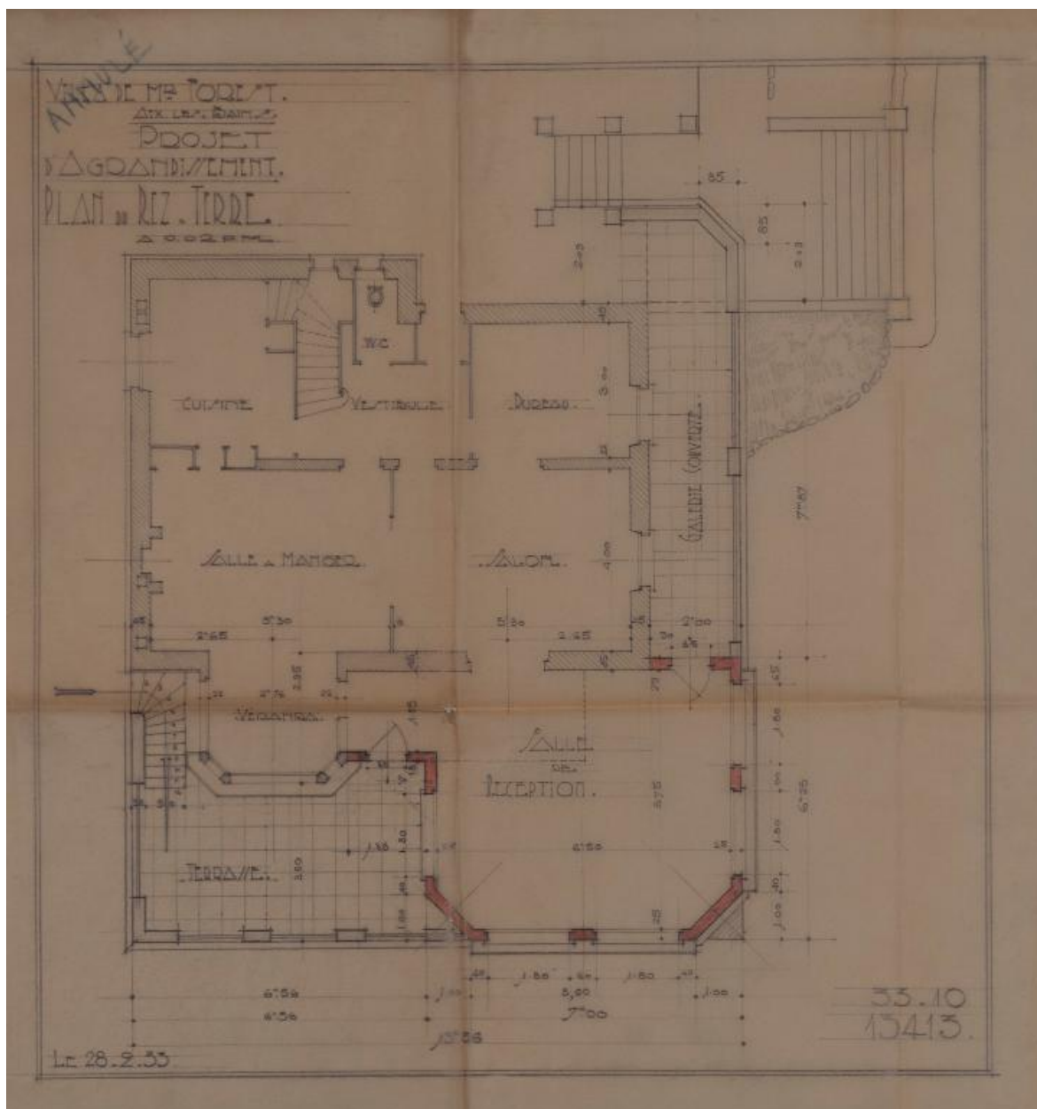
Plan du rez-de-terre, 1933, non réalisé
