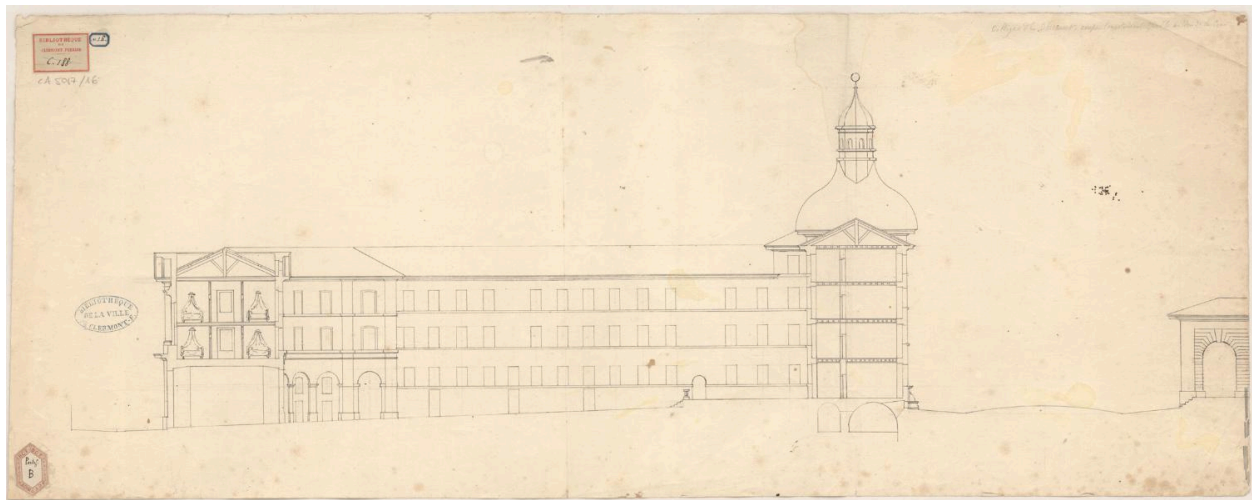
Coupe longitudinale par le milieu de la cour par A. Richier, 1802 (B Patrimoine CAM, CA 5017/16)
