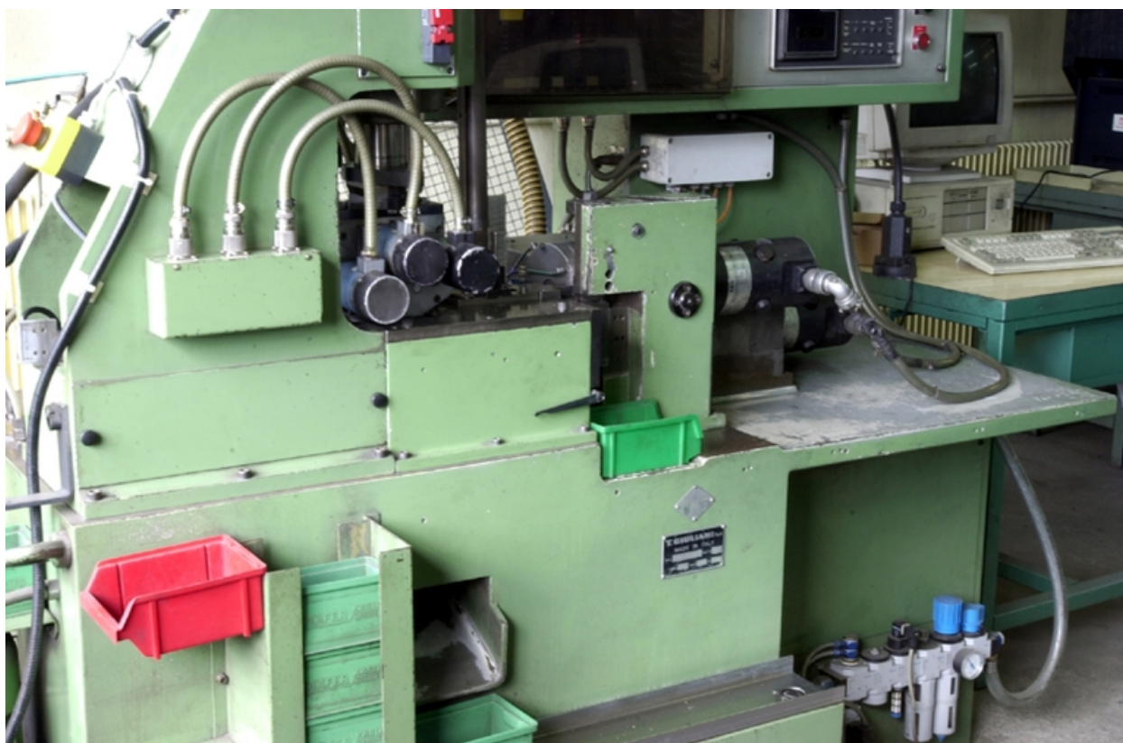
Détail plaque-machine
