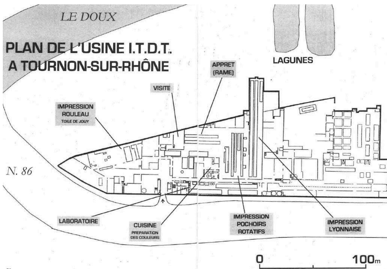
Plan de l'usine ITDI (archive F. Malaval)
