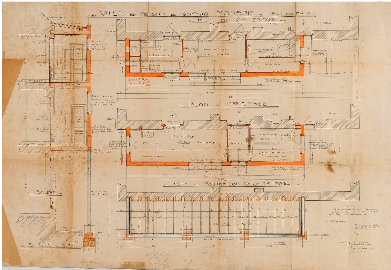
Plans et coupe du corps de porche droit
